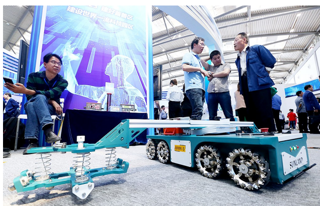
承轨台检测机器人。该机器人在无砟轨道施工过程中,对全线每个承轨台参数进行复测,检测效率是人工测量的2倍以上,大幅度降低垫板更换率,节约人力,缩短工期。 本报记者 鲜康 摄
