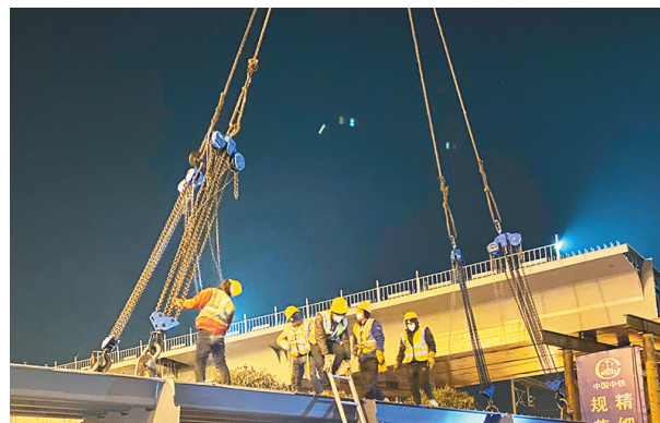
1月1日凌晨,西安北客站枢纽工程SS桥工地,中铁电气化局铁路工程公司建设者在寒冷的冬夜加紧进行箱梁架设。经过7个小时的挑灯夜战,顺利完成了钢箱梁上跨明光路架梁,实现了新年开门红。 □倪树斌 程少为 摄
