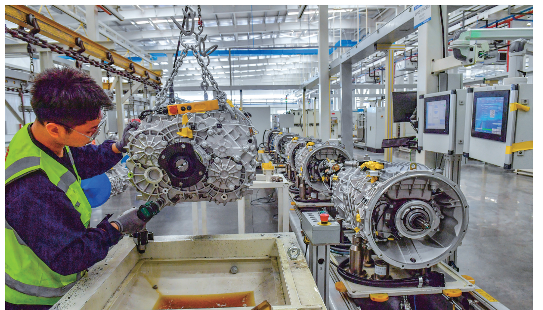
11月1日，在陕西法士特汽车传动集团高智新科技公司智能化生产车间，工人正在有序作业。据了解，该企业今年前10个月销售收入、变速器总成生产同比增长均超52%。袁景智 摄
